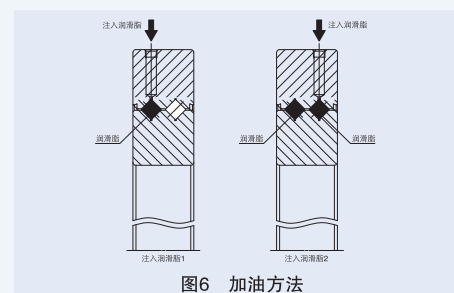
图6 加油方法
